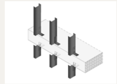
2. Install exterior stud frame
